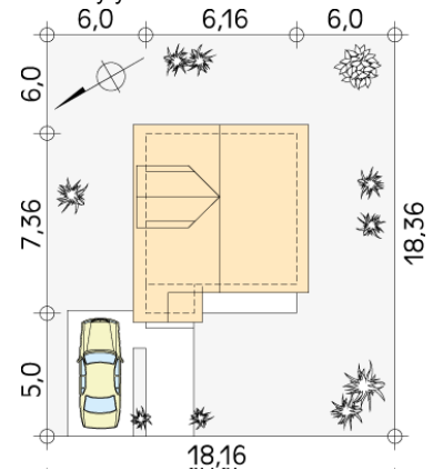
Gabaryty działki:
